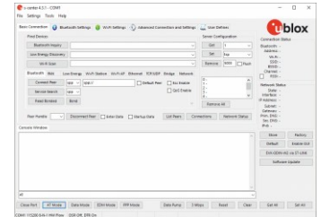
s-center
